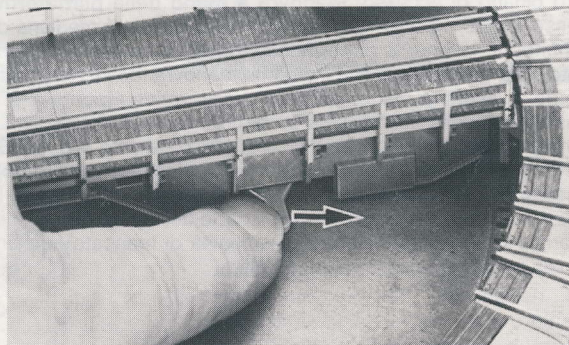
Fig. 12 Sollte trotz Betätigung des Schalters 6910 der Antrieb klemmen oder nicht anlaufen, so ist durch kurzes Drücken des Hebels in Richtung Grubenrand der Antrieb in Betrieb zu setzen. Dieser hält dann nach einer Gleisteilung wieder an.
