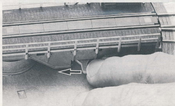
Fig. 11 Gegenüber dem Wärterhaus ist unterhalb der Drehbühne am Antrieb ein Handhebel angebracht. Durch Drücken und gleichzeitiges Halten des Hebels in Richtung Drehbühnenmitte rastet das Antriebsrad aus der Verzahnung der Grube aus und die Drehbühne kann in beliebiger Richtung verstellt werden. Nach Loslassen des Hebels greift das Zahnrad wieder ein. Darauf achten, dass die Gleisteilung der Anschlussgleise mit dem Bühnengleis übereinstimmt.
