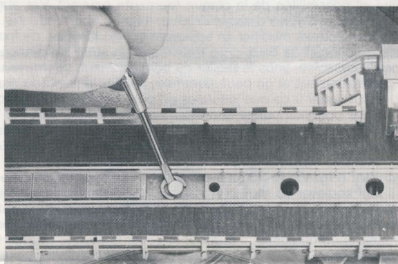
Fig. 15 Läuft die Drehbühne auch nach Betätigung des Handhebels nicht an, muss sie ausgebaut werden. Dazu wird mit einem kleinen Schraubendreher die mittlere Gitterabdeckung zwischen den Schienen der Bühne abgehoben und der Sicherungsring am Drehzapfen entfernt. Vorsicht! Sicherungsring nicht verlieren! Auf jeder Seite der Drehscheibe werden mindestens 6 gegenüberliegende Teilstücke entfernt (siehe Fig. 10). Jetzt kann die Bühne in diesen Ausschnitt gefahren und herausgehoben werden. Die Kontaktbahnen neben dem Drehzapfen und die Kontaktfedern sind zu reinigen.
