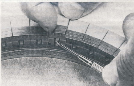
Fig. 9 Mit dem Erweiterungs-Set 9153 kann die Drehscheibe um jeweils drei Gleisanschlüsse erweitert werden.
